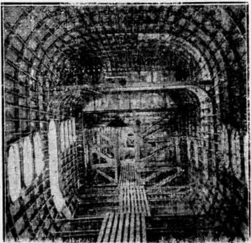
Vista del interior de uno de los nuevos hidroaviones en construcción, mirando contra la proa.
