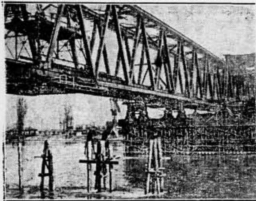
En Bado, sobre el Rhin, se está construyendo un puente de 282 metros de largo. Un solo bloque-pilar, cuyos fundamentos se enterran nueve metros en el lecho del río, sostendrá un peso total de siete mil toneladas. Dispondrá de una triple vía, para trenes, vehículos y peatones.
