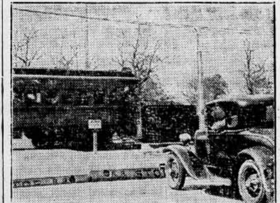
Una Compañía americana de ferrocarriles, ha instalado un aparato en los pasos a nivel, que funciona automáticamente, con señales luminosas durante la noche.
