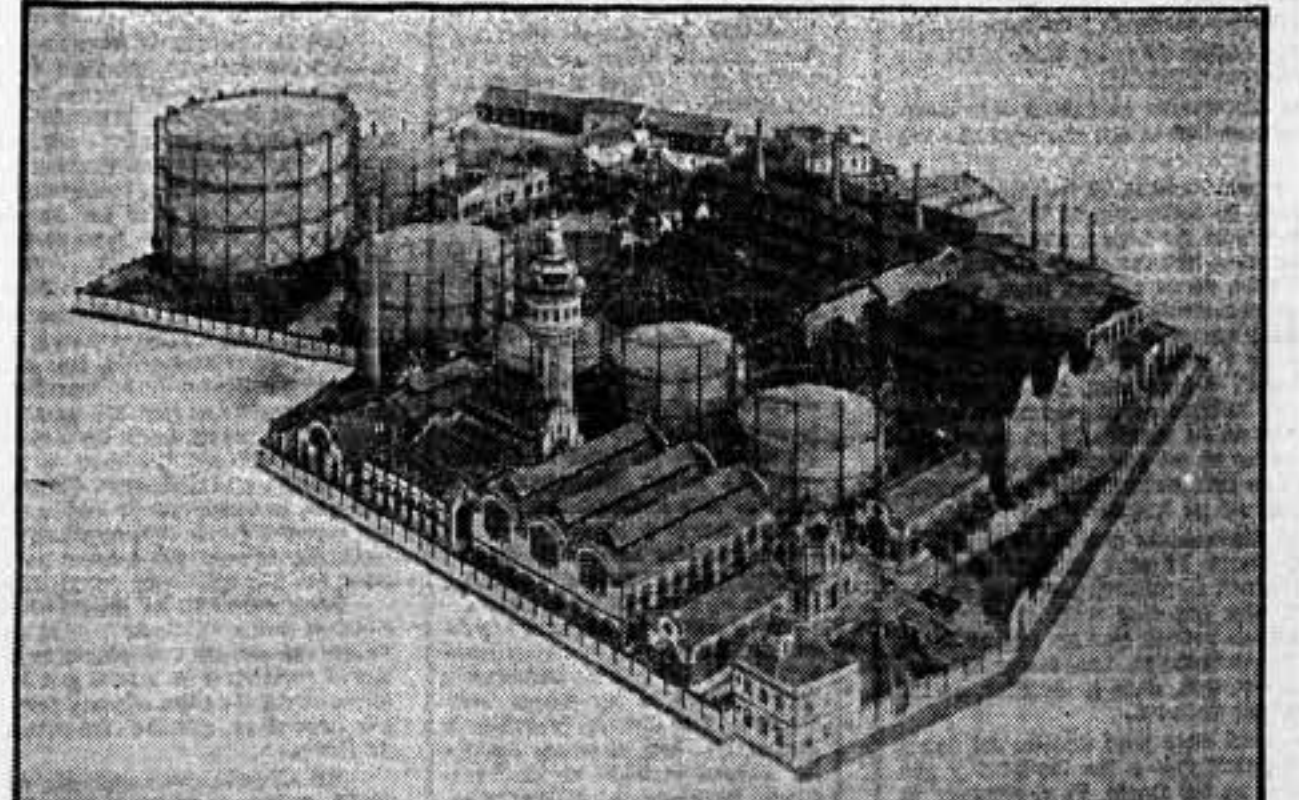
Esta vista general de la fábrica del gas no es otra cosa que la reproducción de una maqueta, en la que se copia a la perfección dicha fábrica. El trabajo de esta maqueta, una de las más notables en su género, ha sido efectuado por un modesto obrero que presta sus servicios en la industria desde hace varios años.
